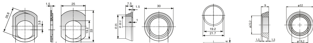
Korokelevy 441345
