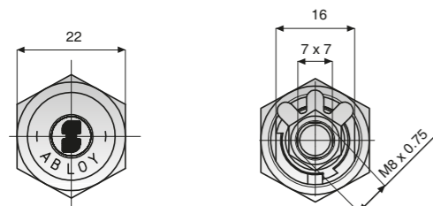
Sylinterin etupinta
